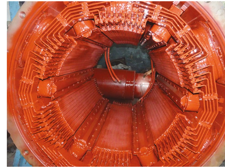
1500 Hp DC mixer motoru bakımı.
