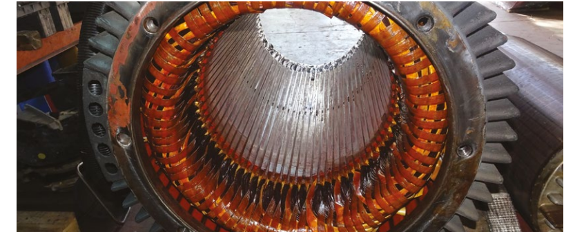
2500 kW atlas copco kompresör motoru sahada yatak değişimi ve laser kaplin ayarı.
